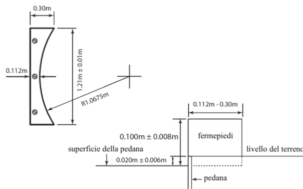
Figura RT 32 a – Pianta del fermapiedi
