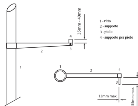
Figura RT 28 b – Salto con l'Asta: supporti per l'asticella (vista dalla zona di caduta e dall'alto)
